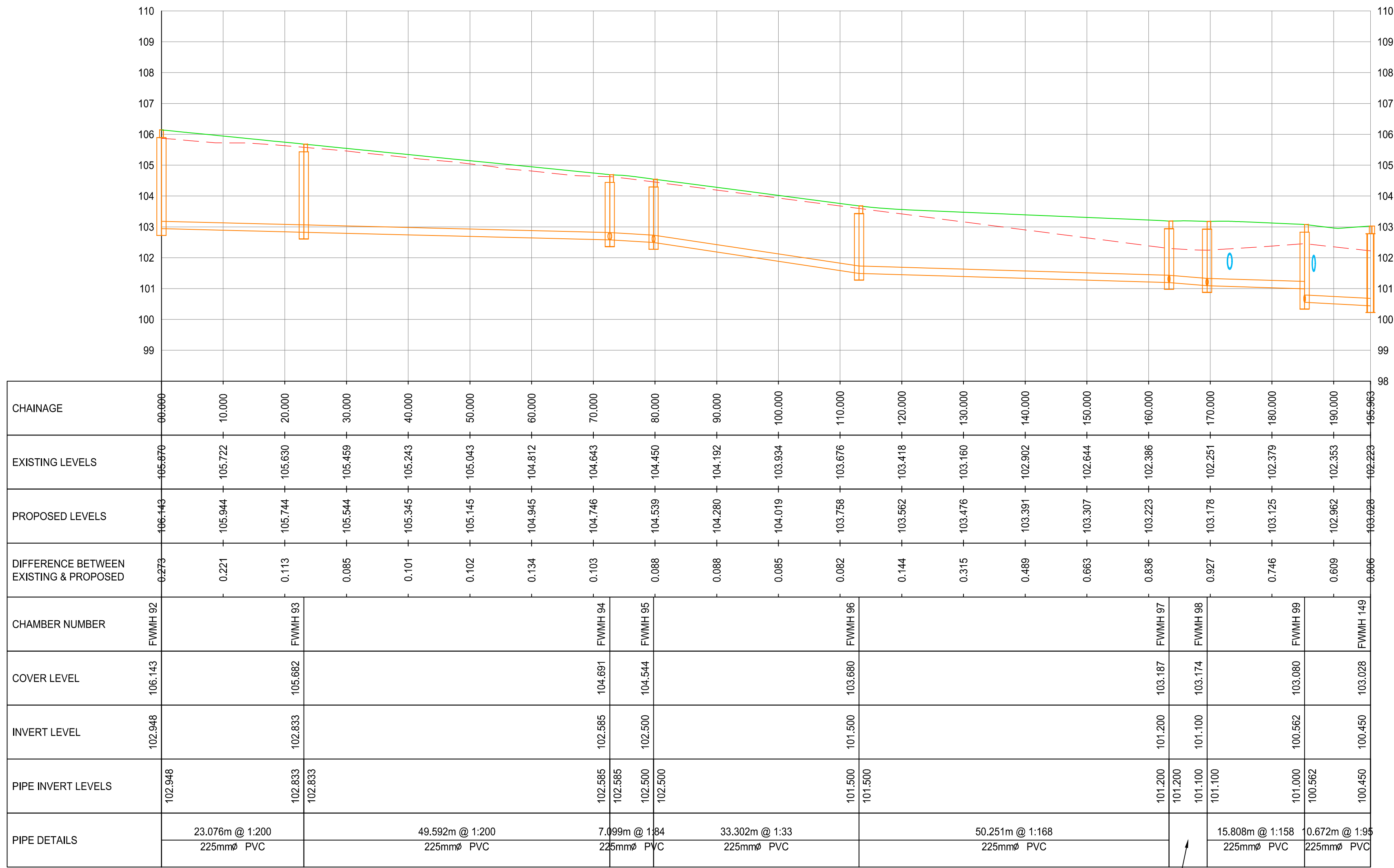
FW 26 SCALE: H 1:500,V 1:100, DATUM: 98.000
