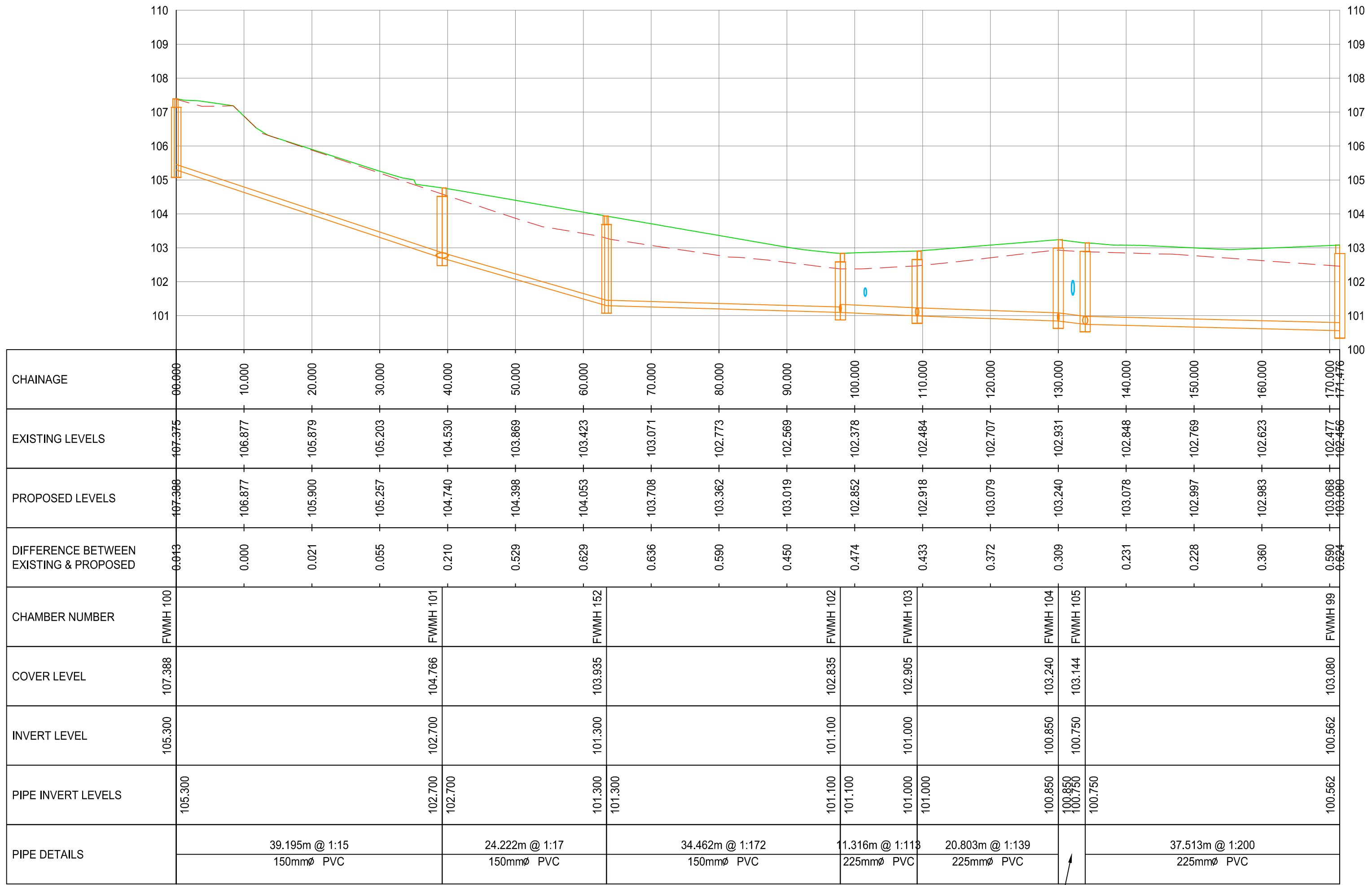
FW 27 SCALE: H 1:500,V 1:100, DATUM: 100.000
